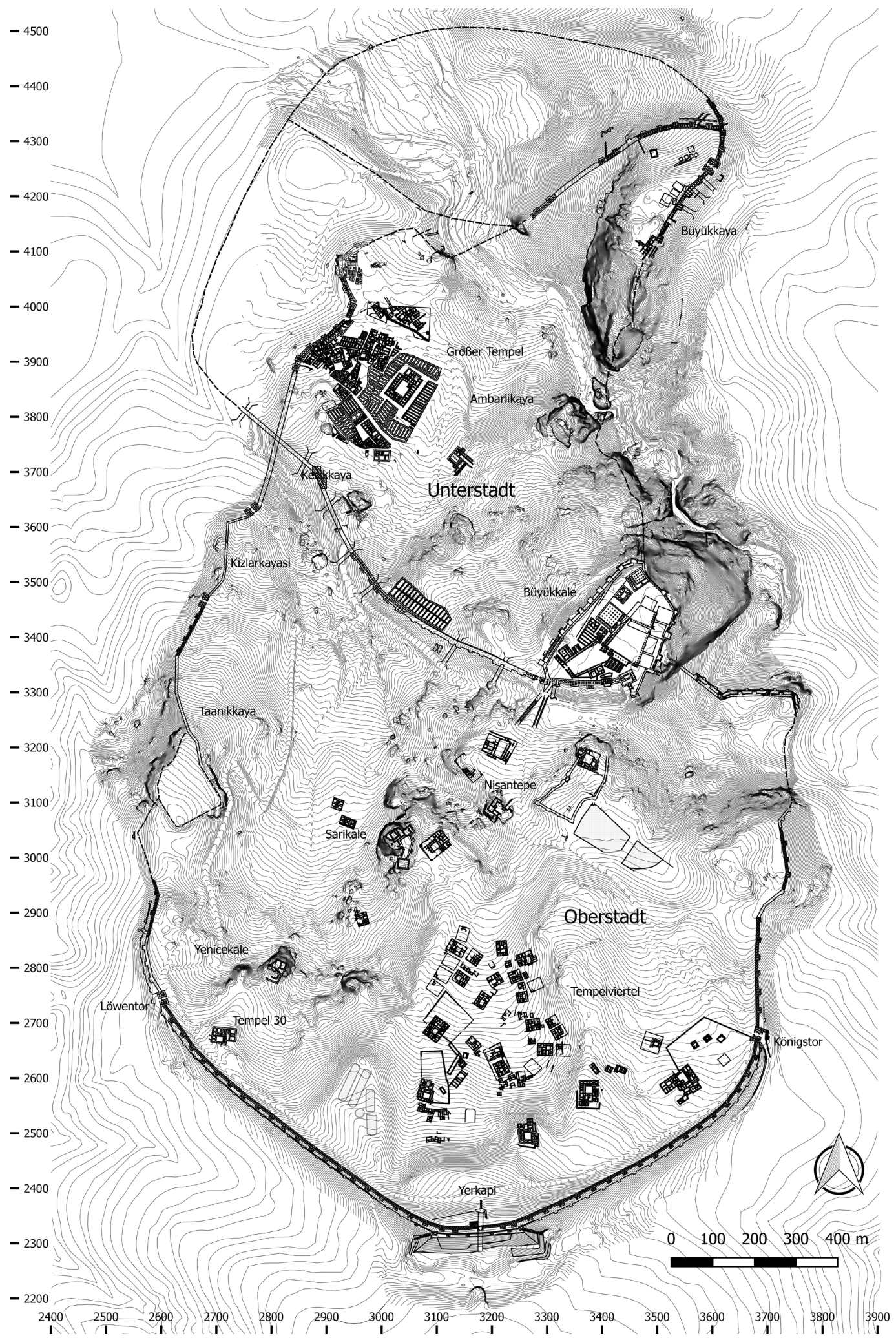
Gesamtplan von Boğazköy-Hattusa zur Großreichszeit (Stand der Grabungen 2010); erstellt von D. Krüger und A. Schachner auf Grundlage der Grabungsdokumentation (Boğazköy-Archiv des DAI, Istanbul)
