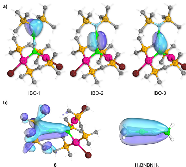
Abbildung 3. a) Ausgewählte IBOs von 6 . b) Die vollständig \pi -delokalisierten MOs von 6 (links, HOMO-30) und H 2 BNBNH 2 (rechts, HOMO-3), die den Cumulen-Charakter ihrer BNBN-Einheit hervorheben.
