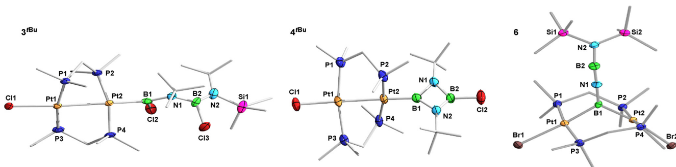
Abbildung 2. Kristallographisch ermittelte Festkörperstrukturen (von links nach rechts) von 3 tBu (nur eines der beiden Moleküle – das mit der geringsten Fehlordnung – in der asymmetrischen Einheit von 3 tBu ist abgebildet), 4 tBu und 6 . [26] Die Ellipsoide repräsentieren 50% der Aufenthaltswahrscheinlichkeit. Die Ellipsoide der Ligandenperipherie und Wasserstoffatome sind nicht abgebildet. Nur die Hauptkomponenten der Fehlorderungen in 3 tBu (terminale B(Cl)NtBu(SiMe_3) -Einheit) und 4 tBu (gesamte (BNtBu)_2Cl -Einheit und ein dmpm-Ligand) sind dargestellt. Aufgrund der Einschränkungen, die bei der Verfeinerung der Fehlorderungen angewendet wurden, können die Strukturparameter von 3 tBu und 4 tBu nicht vollständig diskutiert werden. Ausgewählte Bindungslängen (Å) und -winkel ( ^\circ ) für 3 tBu : Cl1-Pt1 2.4939(13), Pt1-Pt2 2.7067(6), Pt-P 2.2446(14)–2.2651(14), Pt2-B1 2.039(6), B1-N1 1.421(8), Cl1-Pt1-Pt2 172.32(3), P1-Pt2-B1 174.14(16), \Sigma(\angle B1) 360.0(4), Torsionswinkel P1-Pt1-Pt2-P2 -47.8(4) , P3-Pt1-Pt2-P4 -54.32(5) ; für 4 tBu : Cl1-Pt1 2.535(3), Pt1-Pt2 2.7214(7); für 6 : Pt1 \cdots Pt2 3.2397(3), Pt1-B1 2.028(6), Pt2-B1 2.021(6), Pt1-Br1 2.6098(6), Pt2-Br2 2.6363(6), Pt-P 2.2679(15)–2.2913(14), B1-N1 1.396(7), N1-B2 1.237(8), B2-N2 1.388(8), Pt1-B1-Pt2 106.3(3), B1-N1-B2 173.8(6), N1-B2-N2 171.3(7), Torsionswinkel P1-Pt1-Pt2-P2 -12.29(5) , P3-Pt1-Pt2-P4 -23.83(5) .
