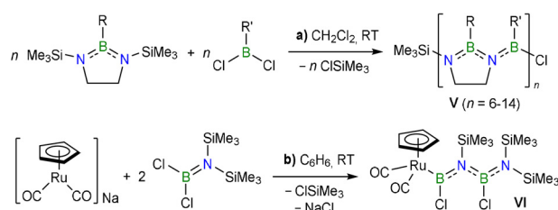
Schema 1. Beispiele für Synthesen von Oligo(iminoboranen) durch B-N-Kupplung über \text{ClSiMe}_3 -Eliminierung.
