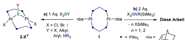
Schema 2. Synthese von Borandiyl-verbrückten Diplatin-A-Frame-Komplexen.
