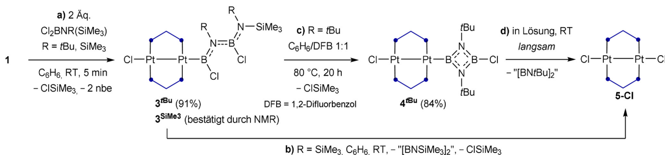
Schema 3. Reaktion von Komplex 1 mit Cl_2BNR(SiMe_3) ( R = tBu, SiMe_3 ). Die isolierten Ausbeuten sind in den Klammern angegeben.
