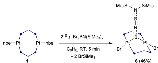
Scheme 4. Reaktion von Komplex 1 mit Br 2 N(SiMe 3 ) 2 . Die isolierten Ausbeuten sind in den Klammern angegeben.
