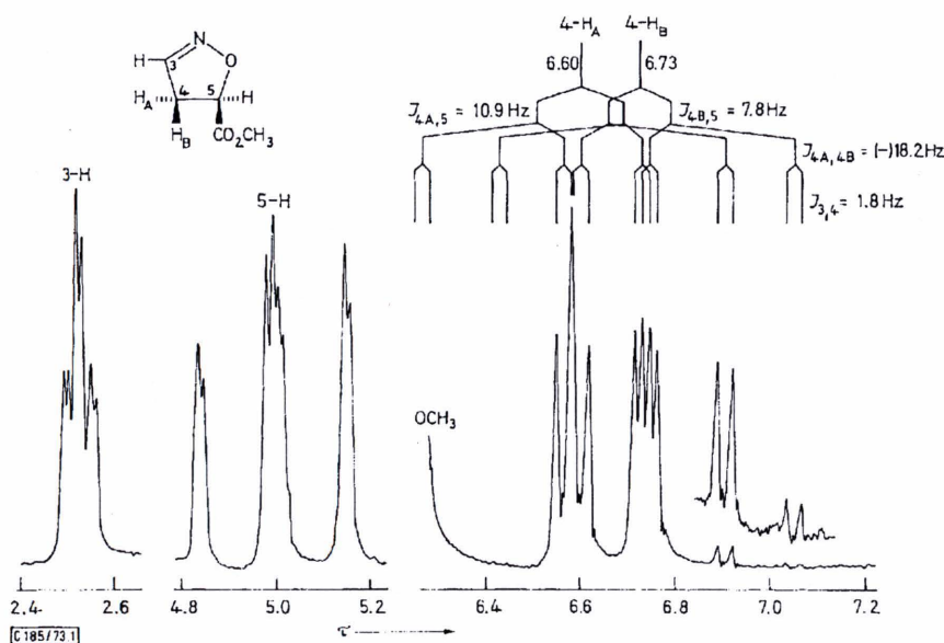
Abb. 1. Ausschnitte aus dem gedehnten NMR-Spektrum des 2-Isoxazolin-5-carbonsäure-methylesters ( 16 ) bei 60 MHz ohne Lösungsmittel mit TMS als internem Standard. Die einzelnen Bandengruppen wurden nicht mit der gleichen Verstärkung gemessen
