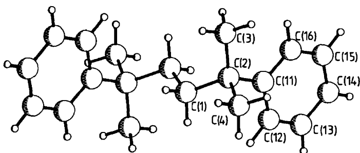
Fig. 4. Molekülstruktur von 4 mit Angabe des Numerierungssystems.
