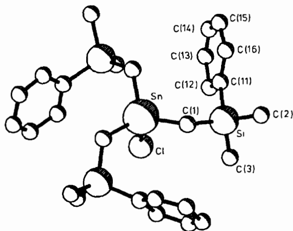
Fig. 2. Molekülstruktur von 1b mit Angabe des Numerierungssystems.
