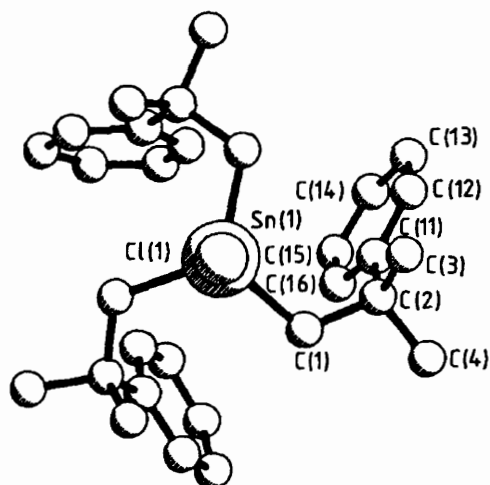
Fig. 1. Molekülstruktur von 1a mit Angabe des Numerierungssystems.
