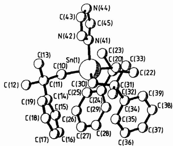
Fig. 3. Molekülstruktur von 2a·0.5H 2 O mit Angabe des Numerierungssystems
