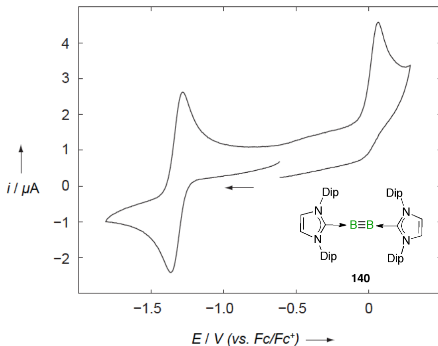
Abbildung 116 Cyclovoltammogramm von [\text{B}_2(\text{IDip})_2] ( 140 ) (0.1 M [(\text{Bu}_4\text{N})\text{PF}_6] / 200 \text{mVs}^{-1} Vorschubgeschwindigkeit)
