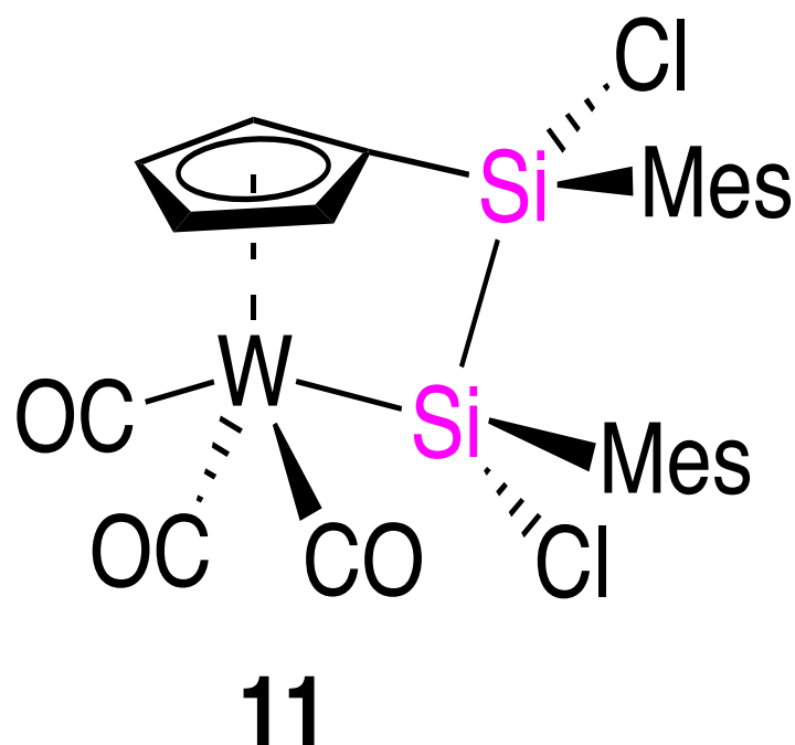
Abbildung 7 Synthesestrategien für ansa -Sandwichverbindungen.
