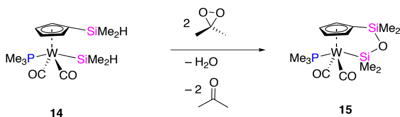
Abbildung 10. Synthese von ansa -Halbsandwichverbindungen der sechsten Gruppe durch intramolekulare C–H Aktivierung eines Fluorenylliganden.
