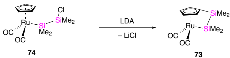
Abbildung 54 Synthese von [\{\kappa^1\text{-SiMe}_2\text{SiMe}_2(\eta^5\text{-C}_5\text{H}_4)\}(\text{CO})_2\text{Ru}] ( 73 ) durch baseninduzierte Migration.
