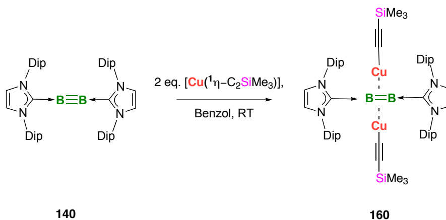
Abbildung 131 Reaktion von zwei Äquivalenten [\text{Cu}(\eta^1\text{-C}_2\text{SiMe}_3)] sowie vier mit [\text{B}_2(\text{IDip})_2] ( 140 ).
