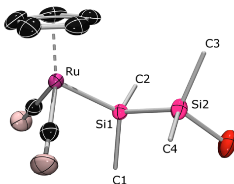
Abbildung 53 Molekülstruktur von [(\eta^5\text{-C}_5\text{H}_5)\text{Ru}(\text{CO})_2(\text{SiMe}_2\text{SiMe}_2\text{Cl})] ( 74 ). Die thermischen Ellipsoide sind auf dem 50%-Wahrscheinlichkeitsniveau abgebildet. Die Wasserstoffatome sowie die Ellipsoide der Methylgruppen sind aus Gründen der Übersichtlichkeit nicht dargestellt. Ausgewählte Bindungslängen [Å] und -winkel [°]: Ru–Si1 2.4170(7), Si1–Si2 2.3368(8), Si2–Cl 2.098(1), Ru–Si1–C2 112.58(8), Ru–Si1–Si2 111.02(3), C1–Si1–C2 106.1(1), Ru–Si1–C1 114.47(7), Si1–Si2–Cl 106.46(3), C3–Si2–Cl 104.8(1), C4–Si2–Cl 105.9(1), C3–Si2–C4 109.9(1).
