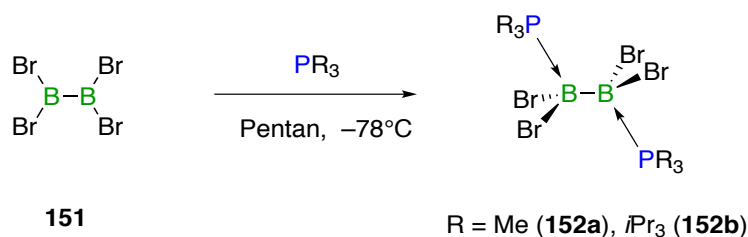
Abbildung 67 Versuchte Darstellung von [\{\kappa^1\text{-Sn}t\text{Bu}_2\text{Sn}t\text{Bu}_2(\eta^5\text{-C}_5\text{H}_4)\}(\text{CO})\text{Ni}] ( 88 ).
