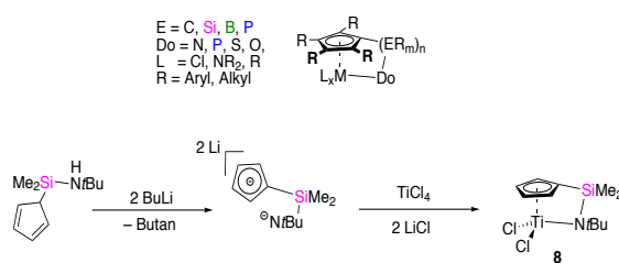
Abbildung 3 Komplexe mit Pianostuhl [20] bzw. Melkschemelgeometrie. [21]
