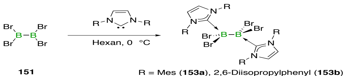
Abbildung 70 Synthese der borverbrückten ansa -Halbsandwichkomplexe 47 und 48 , sowie Darstellung des Monophosphankomplexes 56 .
