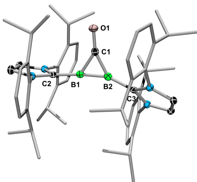
Abbildung 120 Molekülstruktur von [B_2COIDip_2] 158 . Die Wasserstoffatome und die Kohlenstoffatome der Phenylringe und der Isopropyl gruppen sind aus Gründen der Übersichtlichkeit nicht dargestellt. Die thermischen Ellipsoide sind auf dem 50%-Wahrscheinlichkeitsniveau abgebildet. Ausgewählte Bindungslängen [Å] und -winkel [°]: B1–B2 1.549(3), C1–B1 1.565(3), C1–B2, 1.485(3), O1–C1 1.249(2), O1–C1–B2 155.38(17), O1–C1–B1 143.62(16), B2–C1–B1 61.00(13).
