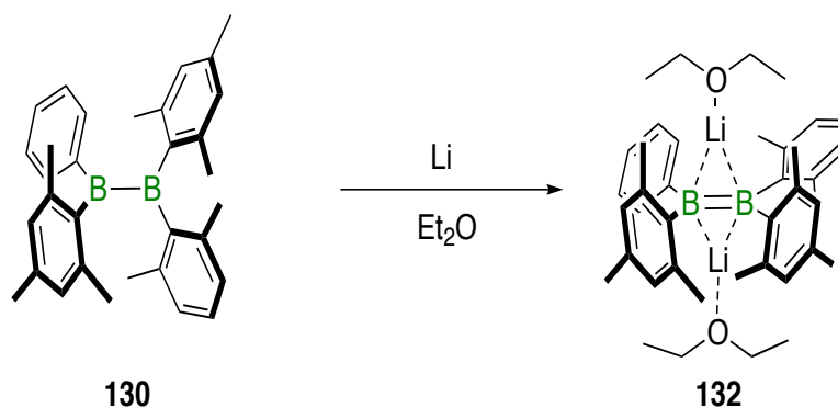
Abbildung 57 Synthese der Chalkogeninsertionsprodukte.
