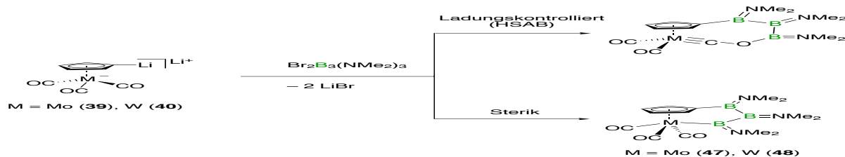
Abbildung 16 Synthese des 1,3-Tristanna-ansa-Halbsandwichkomplexes 17 durch Stannylenewanderung.
