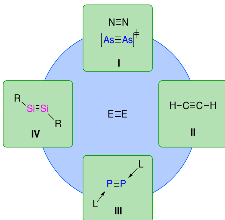
Abbildung 44 Synthesestrategien zu \text{M}[(\eta^5\text{-C}_5\text{H}_4)\{(\text{CO})_2\text{Os}] ( 62 ).
