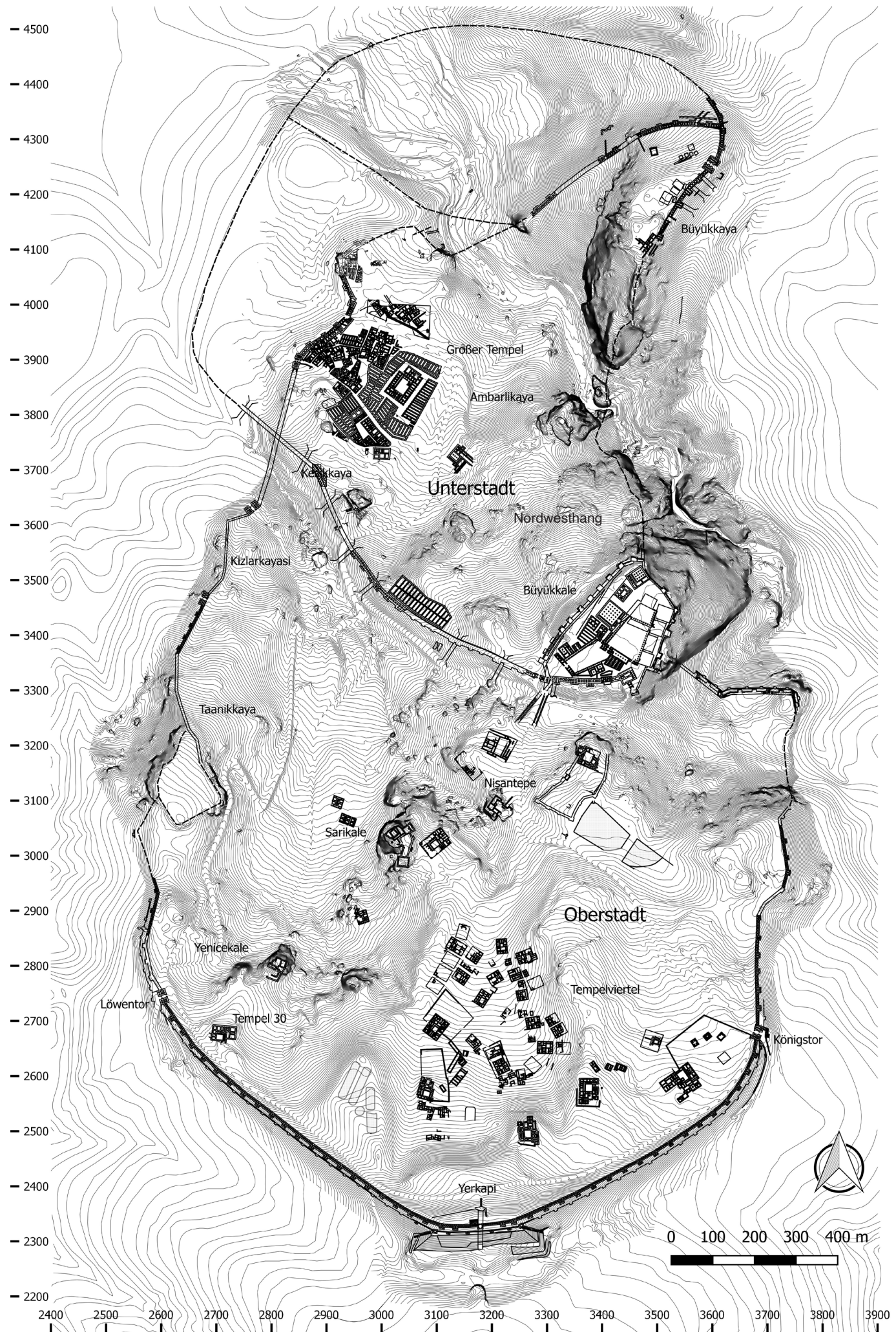
Gesamtplan von Boğazköy-Hattusa zur Großreichszeit (Stand der Grabungen 2018); erstellt von D. Krüger und A. Schachner auf Grundlage der Grabungsdokumentation (Boğazköy-Archiv des DAI, Istanbul)
