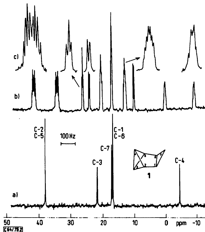
Abb. 2. ^{13}\text{C} -NMR-Spektrum von Tetracyclo[4.1.0.0 2.4 .0 3.5 ]heptan (1) bei 22.63 MHz in [\text{D}_6] -Benzol: a) breitbandenkoppeltes Spektrum, b) protonenkoppeltes Spektrum, c) gedehnte Ausschnitte aus b, wobei die Spektrumamplitude nicht für alle Banden gleich ist
