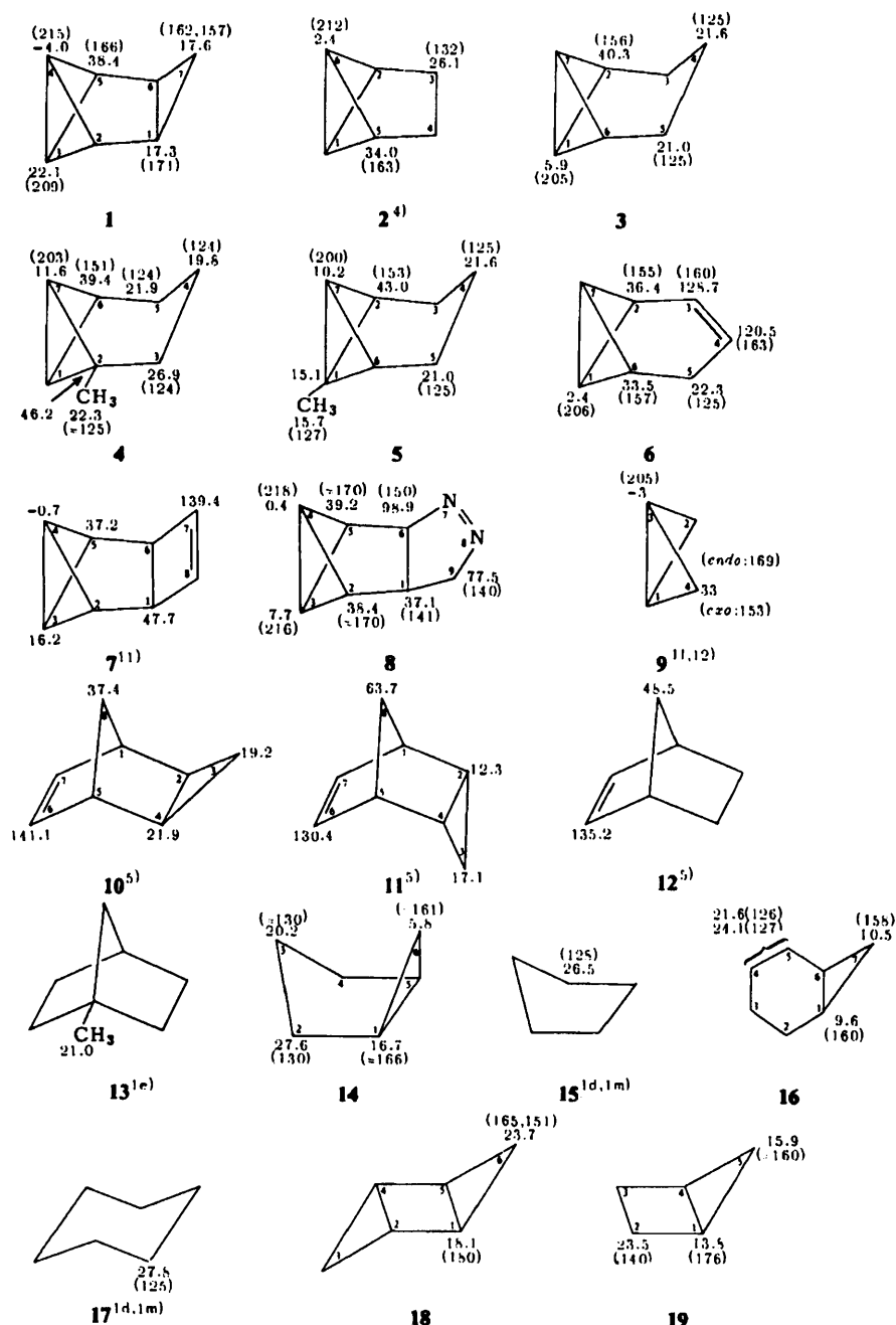
Schema 1. ^{13}\text{C} -Chemische Verschiebungen (in ppm feldabwärts von Tetramethylsilan) und ^{13}\text{C} -H-Kopplungskonstanten (in Hertz, Zahlen in Klammern) von einigen Bicyclo[n.1.0]kohlenwasserstoffen und Vergleichsverbindungen. Die Literaturzitate beziehen sich auf das publizierte ^{13}\text{C} -NMR-Spektrum der betreffenden Substanz.
